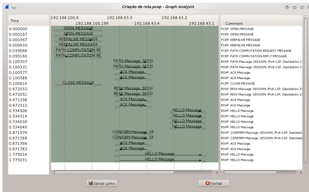
Figura 9. Captura do tráfego das mensagens de controle para criação de um caminho
